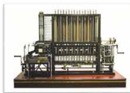
Рис. 1. Машина Беббіджа
