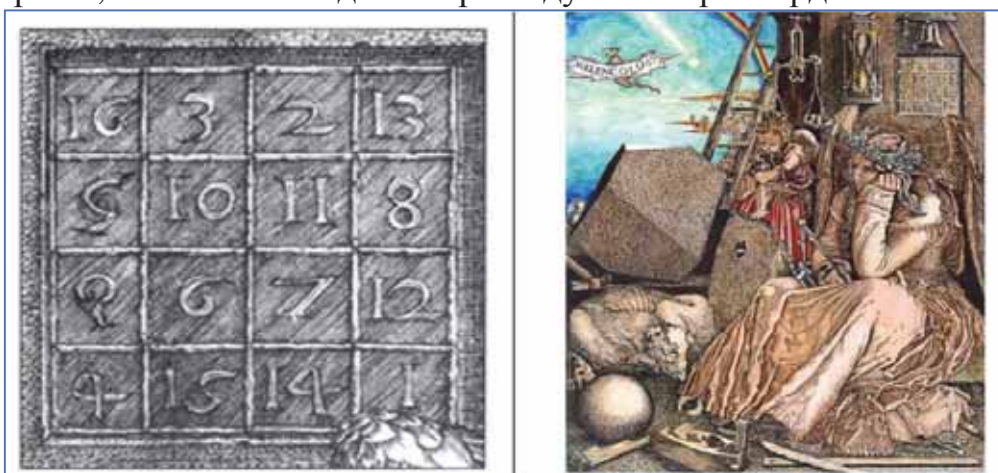
Рис. 2. Магічні квадрати
