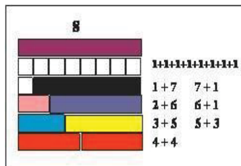
Рис. 7. Склад числа 8.
